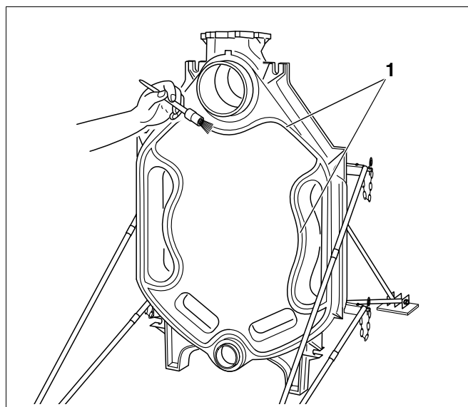
Рис. 15 Смазка пазов для уплотнений адгезионным составом
