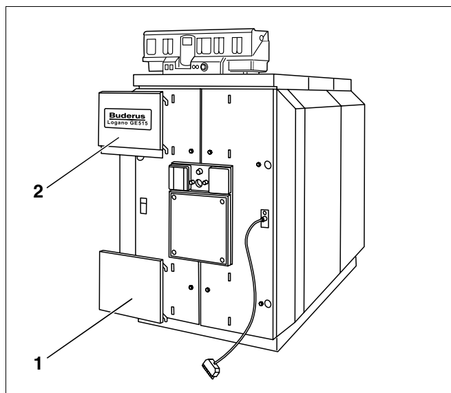
Рис. 58 Установка экранов дверцы горелки
